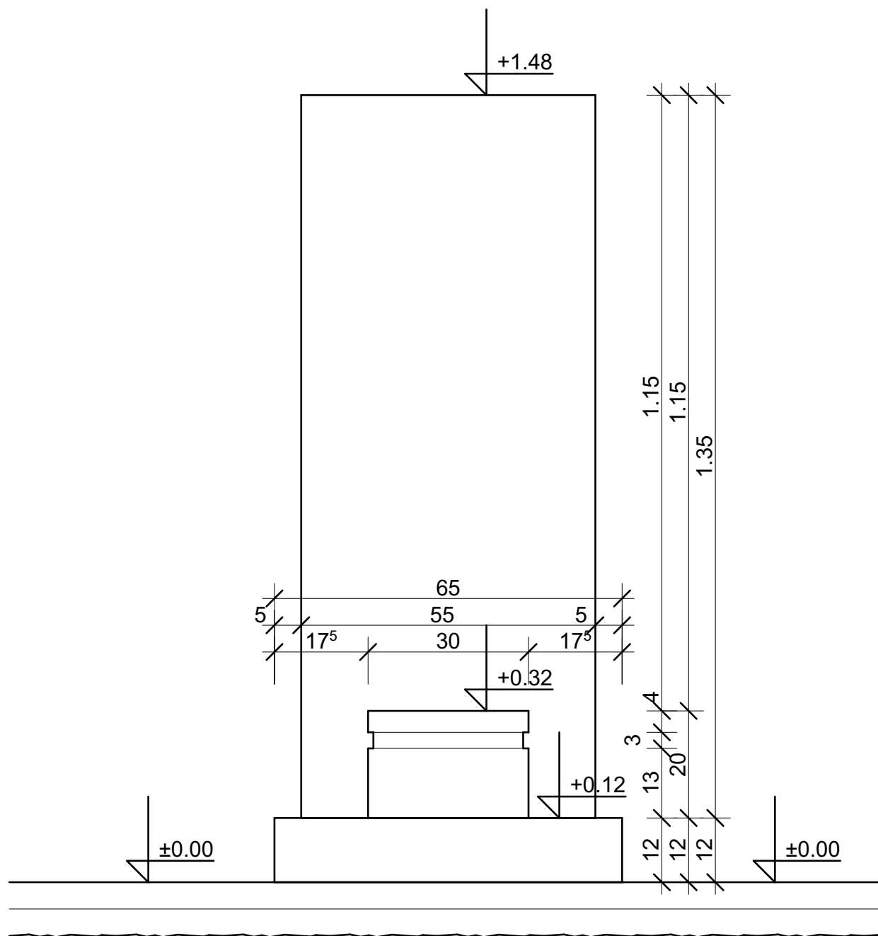
ИЗГЛЕД
