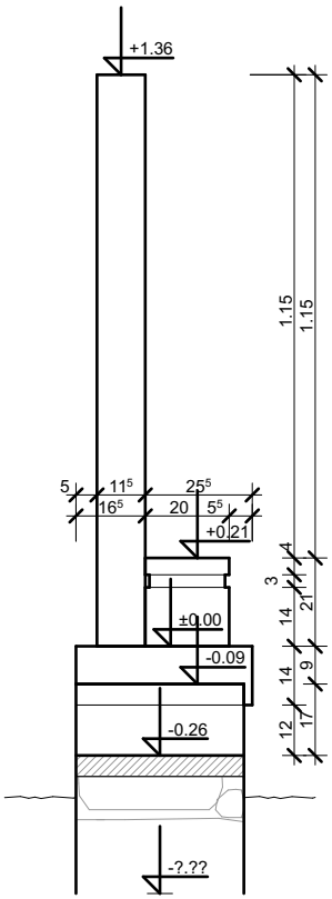
ПРЕСЕК / ИЗГЛЕД
