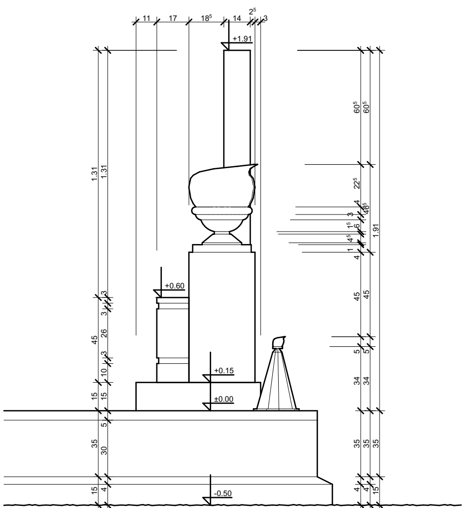
БОЧНИ ИЗГЛЕД
