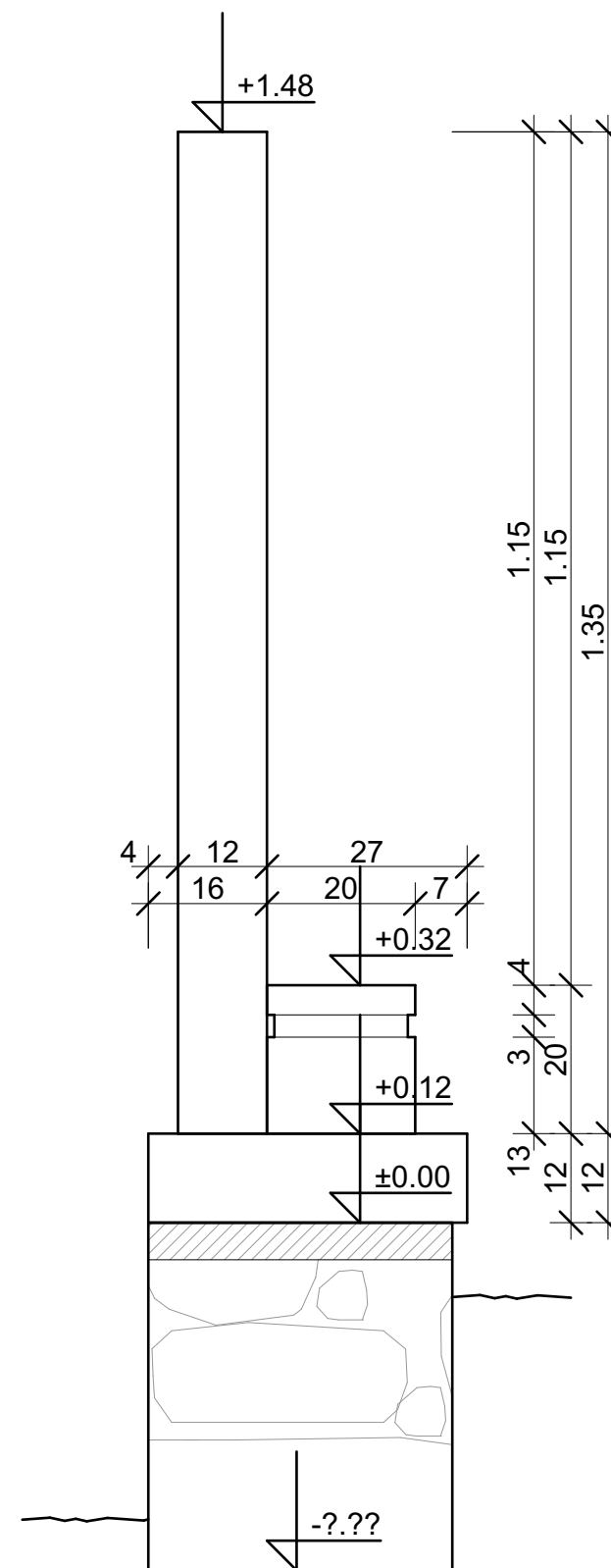
ПРЕСЕК / ИЗГЛЕД
