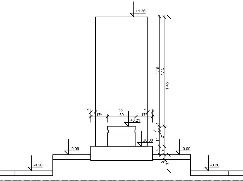
ИЗГЛЕД
